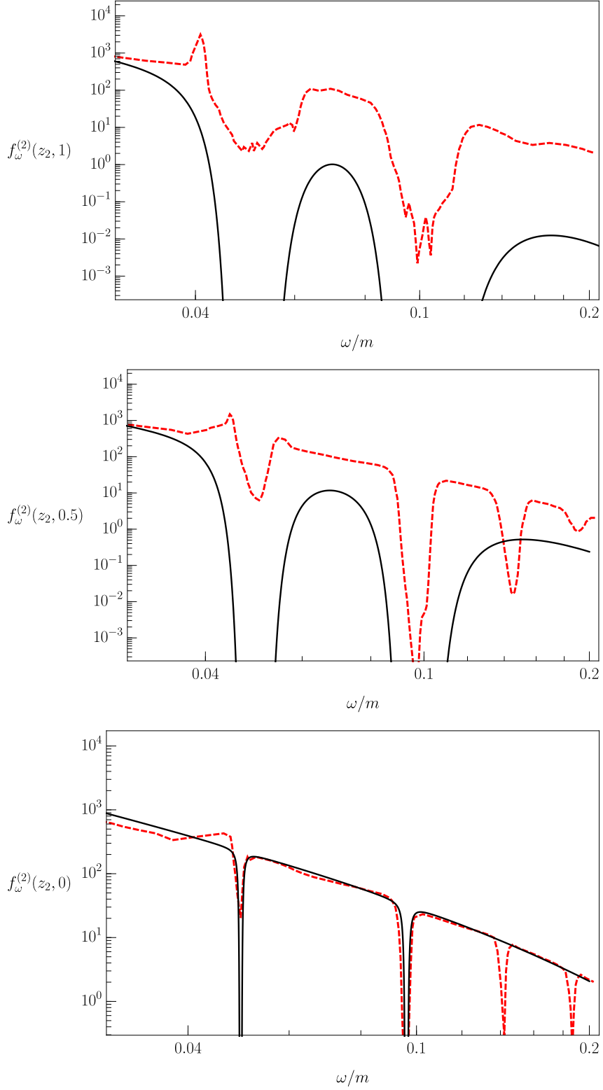
Рис. 4: Функция распределения фотона моды 2 при магнитном поле B = 0.05B_e и температуре T = 3 кэВ, для углов \theta = 0 ( x = 0 ), \theta = \pi/3 ( x = 0.5 ) и \theta = \pi/2 ( x = 1 ) между направлением импульса начального фотона и направлением магнитного поля, а также оптической толщины \tau_2 = 3 \times 10^{-3} . Штриховая линия соответствует результатам, полученным в работе [25], а сплошная линия – дельта-функциональному приближению (30).
