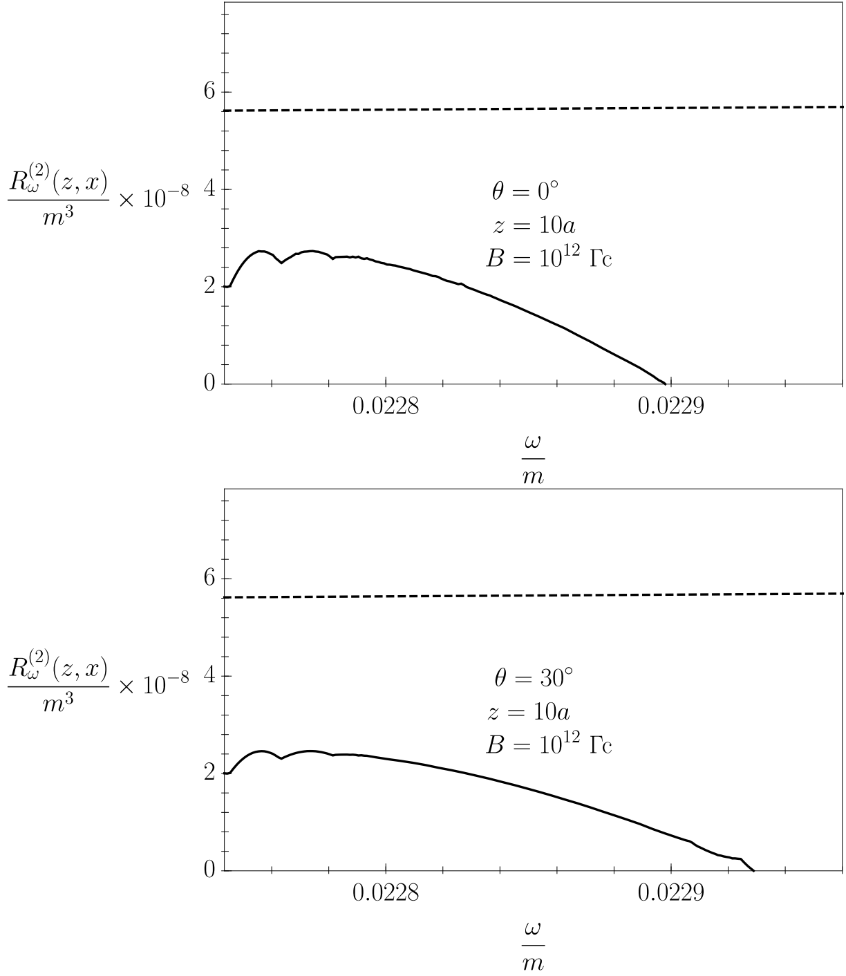
Рис. 8: Спектральная плотность (48) моды 2 с учетом резонансного комптоновского процесса. Штриховая линия – спектральная плотность чернотельного излучения (52)
