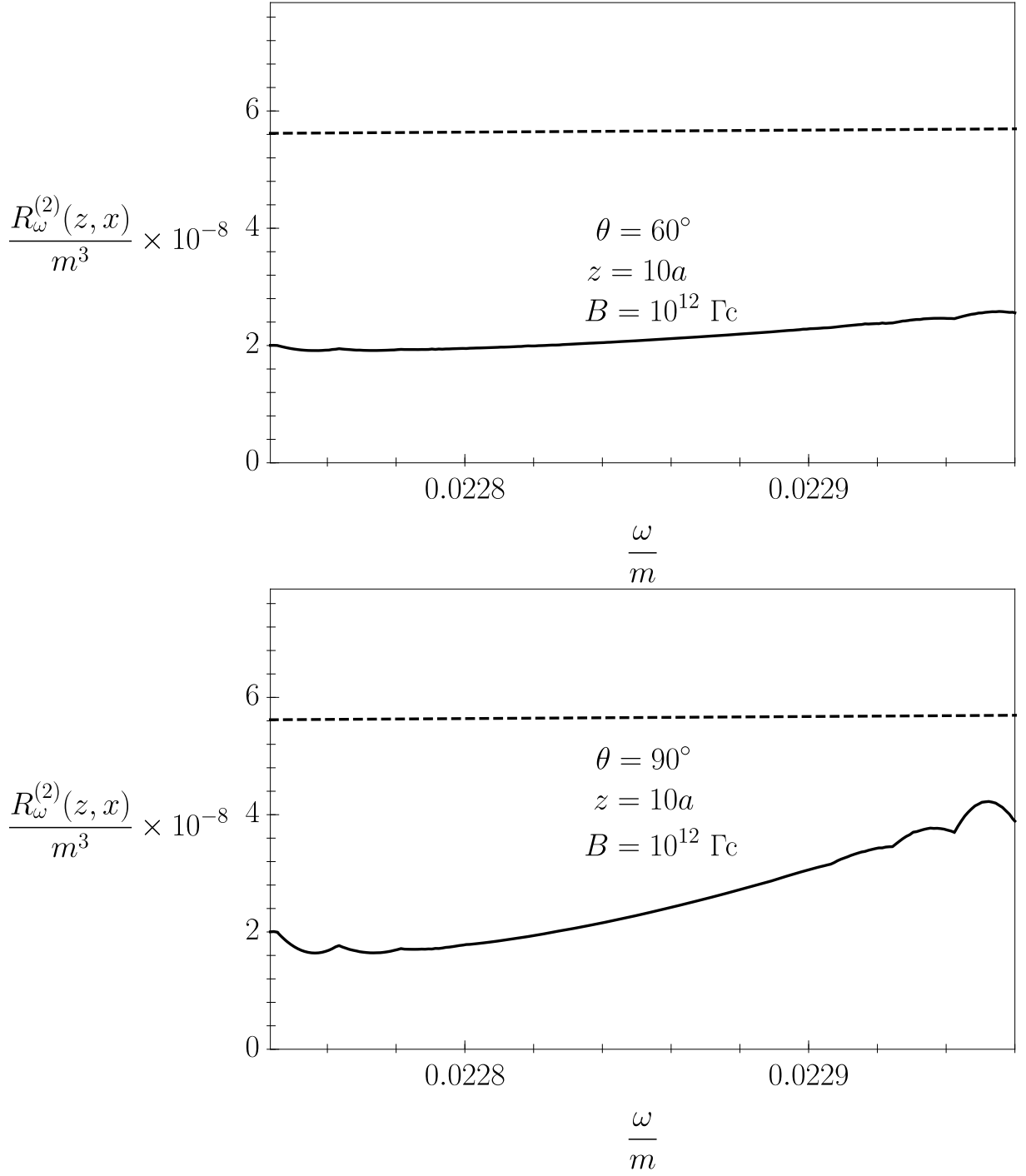
Рис. 9: Спектральная плотность (48) моды 2 с учетом резонансного комптоновского процесса. Штриховая линия – спектральная плотность чернотельного излучения (52)
