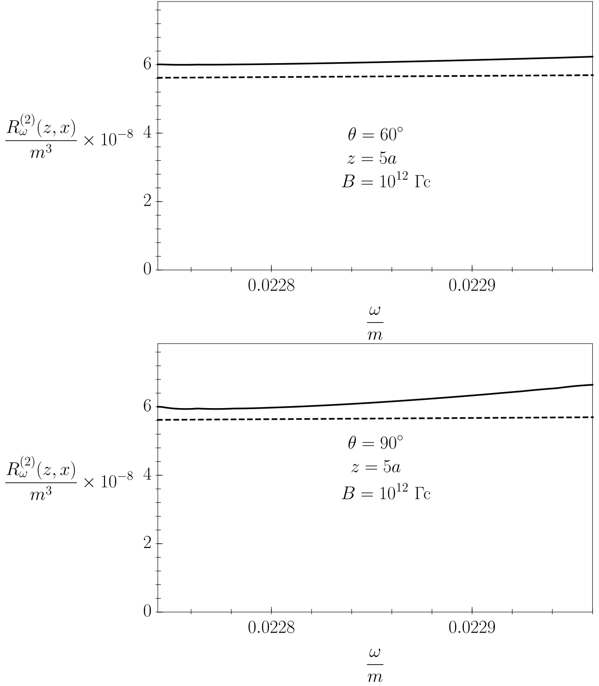
Рис. 7: Спектральная плотность (48) моды 2 с учетом резонансного комптоновского процесса. Штриховая линия – спектральная плотность чернотельного излучения (52)
