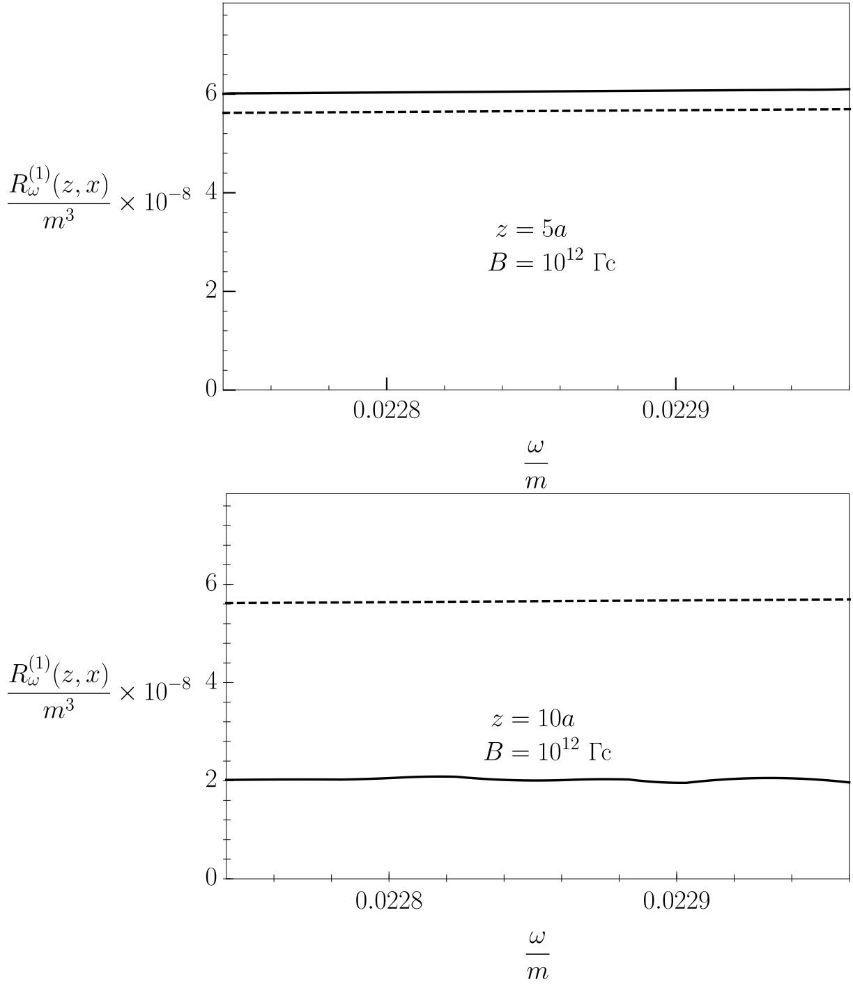
Рис. 5: Спектральная плотность (48) моды 1 с учетом резонансного комптоновского процесса для произвольного угла между направлением импульса начального фотона и направлением магнитного поля. Штриховая линия – спектральная плотность чернотельного излучения (52).
