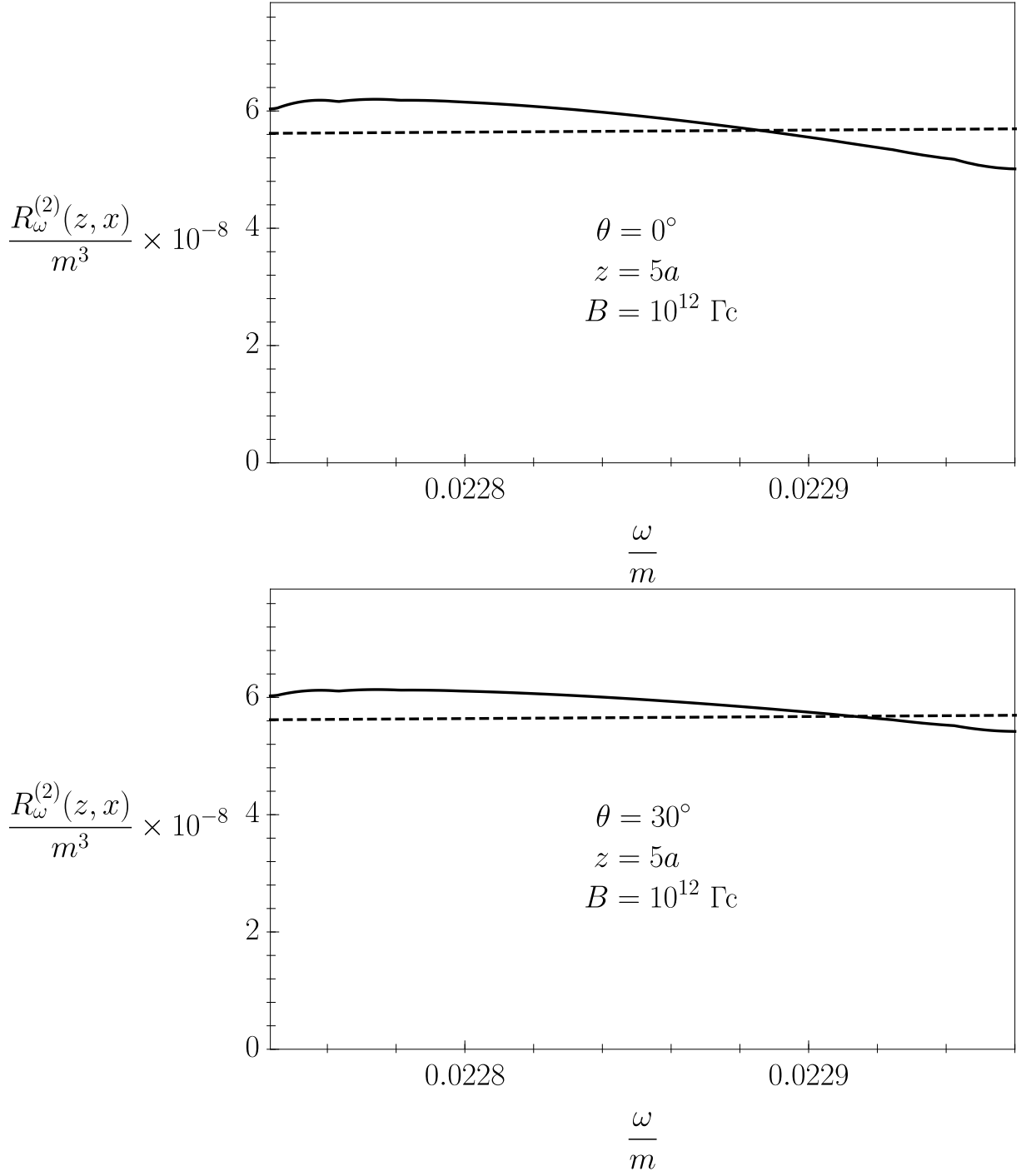
Рис. 6: Спектральная плотность (48) моды 2 с учетом резонансного комптоновского процесса. Штриховая линия – спектральная плотность чернотельного излучения (52)
